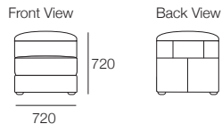
720R Module 720 FIXED Module Headrest Down
